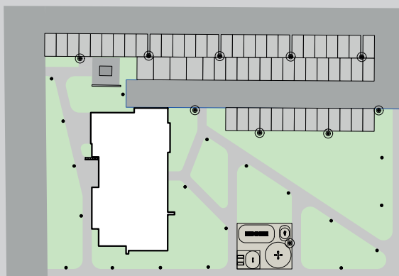
PLAN SYTUACYJNY
